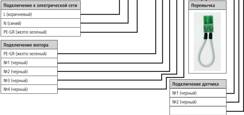
Рисунок 7. Схема подключения платы с конденсатором Uno
