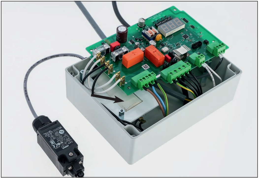
Abbildung 8: Platine in Steuerungsgehäuse (Kondensator hinter der Platine)
