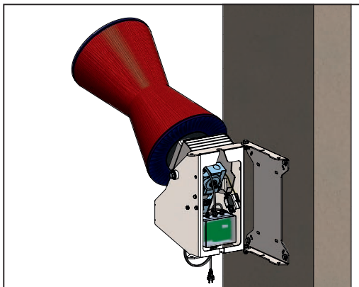
Rysunek 5: Odchylanie maszyny od podstawy
