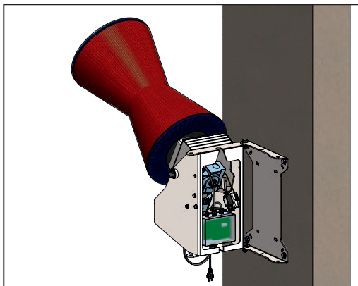
Illustration 5 : Écarter la machine de la base par pivotement
