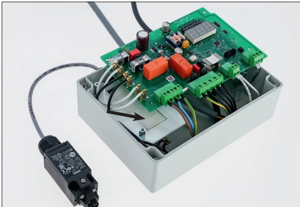
Kuva 8: Piirilevy ohjausyksikön kotelossa (kondensaattori piirilevyn takana)
