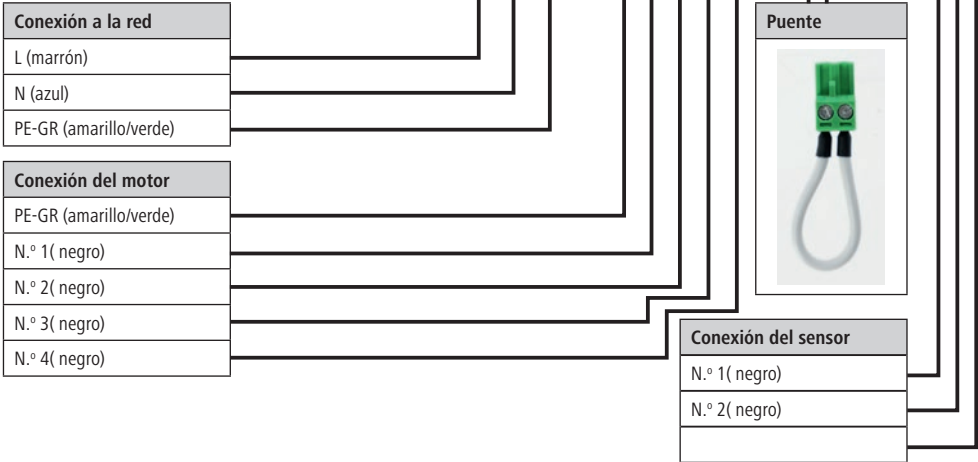
Figura 7: Esquema de conexiones del circuito impreso con condensador (Uno)
