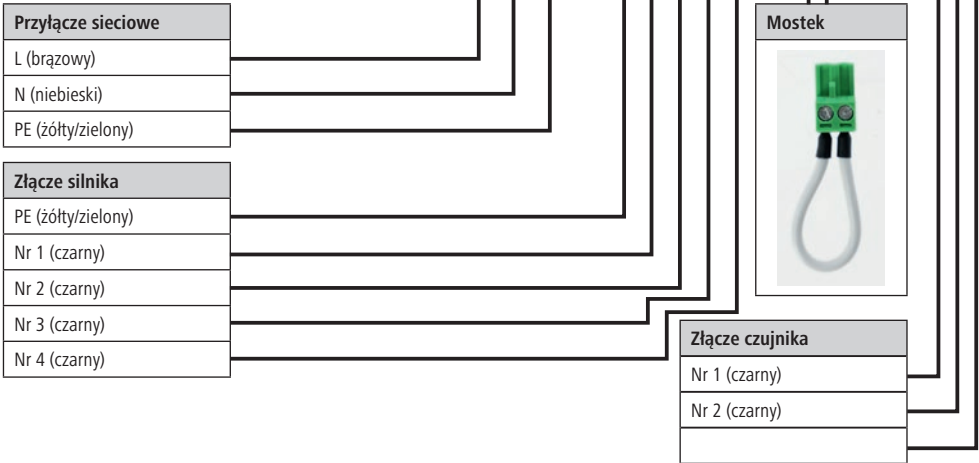
Rysunek 7: Schemat podłączenia płyty z kondensatorem – Uno
