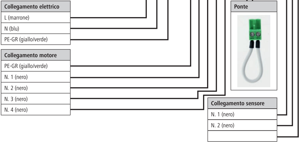
Figura 7: Schema di collegamento della scheda con condensatore - Uno
