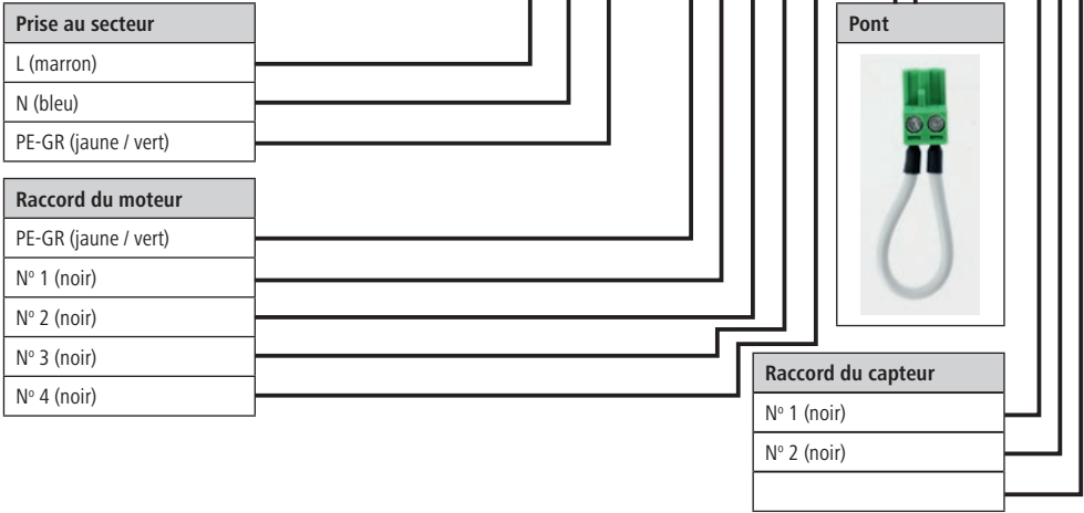
Illustration 7 : Schéma de raccordement de la carte avec le condensateur – Uno
