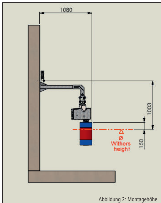
Abbildung 2: Montagehöhe
