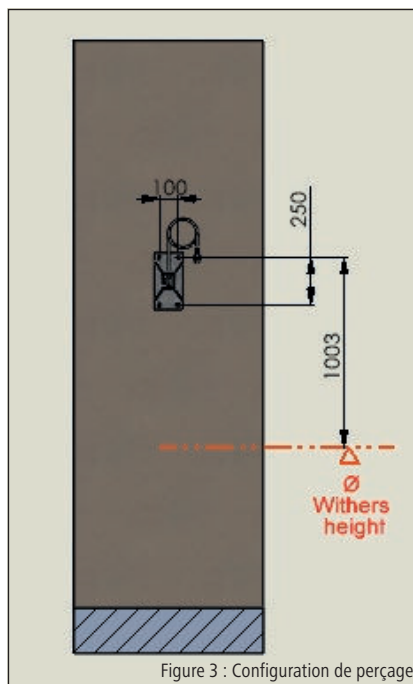
Figure 3 : Configuration de perçage
