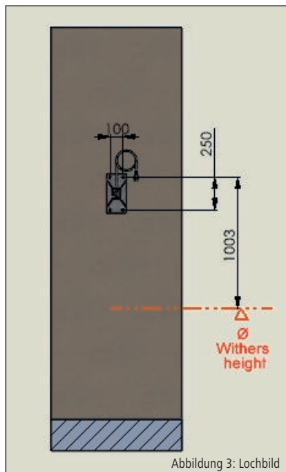
Abbildung 3: Lochbild
