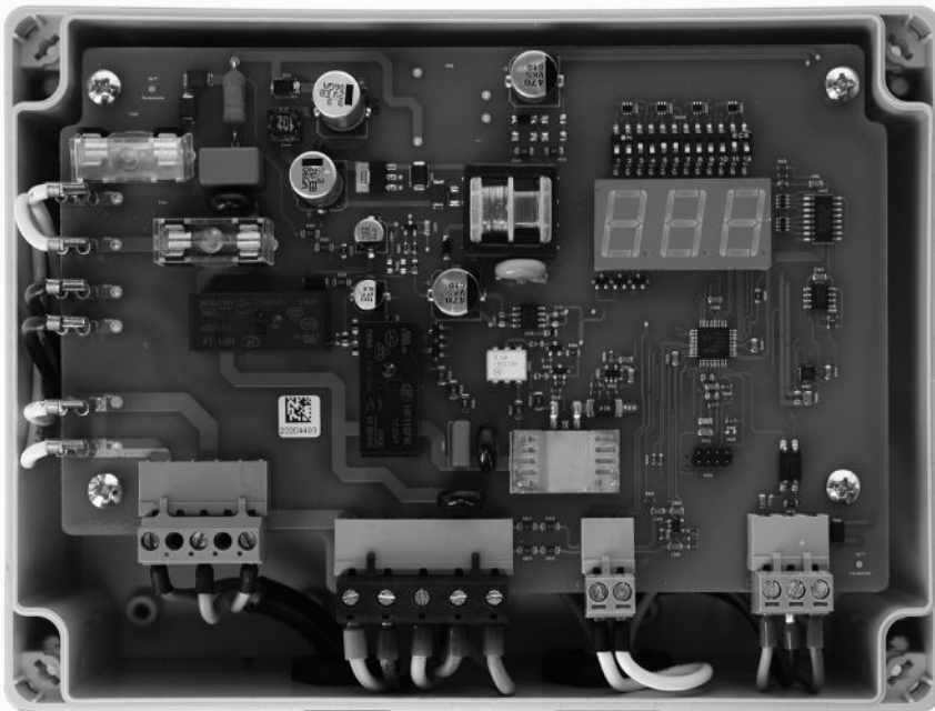
Abbildung 9: Platine in Steuerungsgehäuse (Kondensator hinter der Platine)
