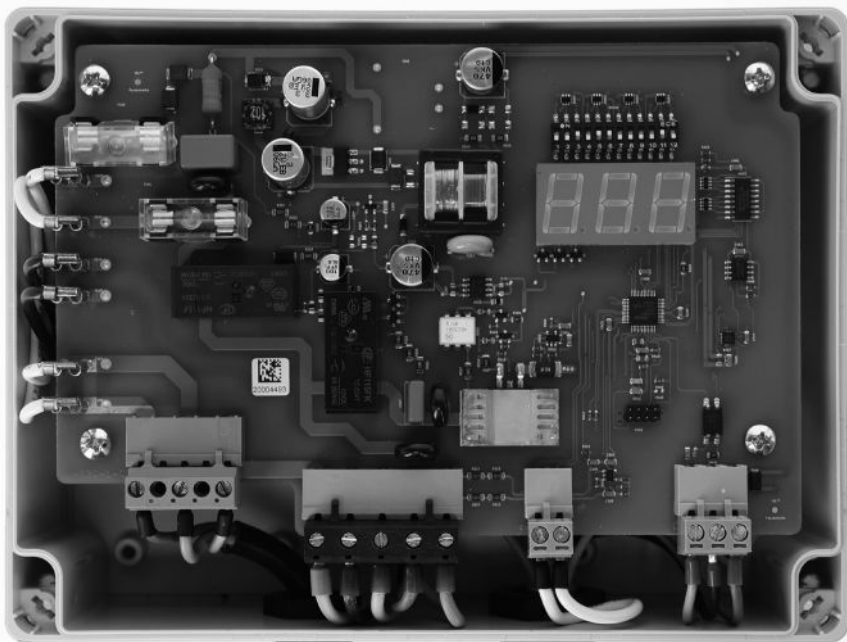
Kuva 9: Piirilevy ohjausyksikön kotelossa (kondensaattori piirilevyn takana)
