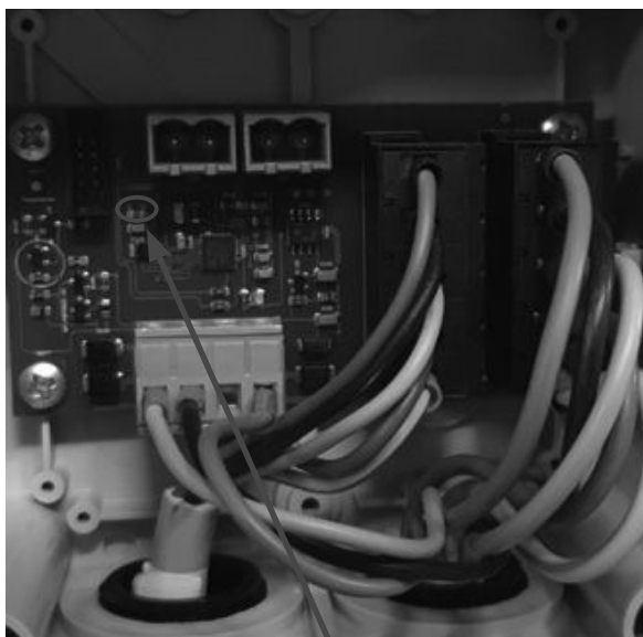
Рисунок 11. Плата датчиков
