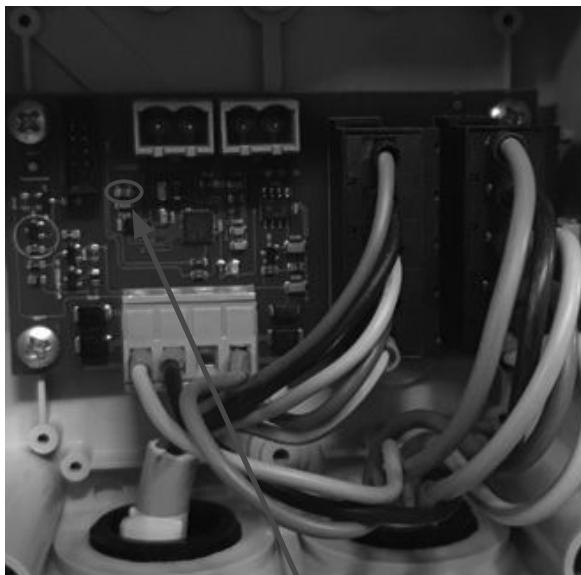
Afbeelding 11: Sensorprintplaat
