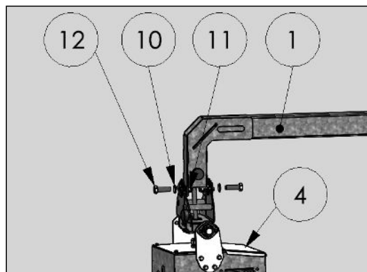
Abbildung 4: Montage Bürste mit Antriebseinheit
